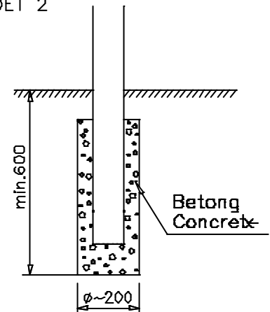
DET 2
