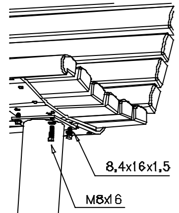
DET 2
